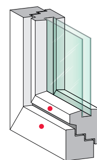
halbfächenversetzt
